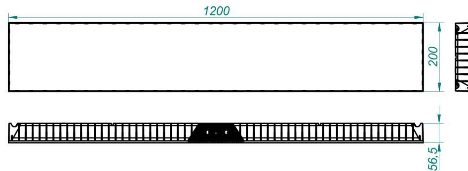
Рисунок 16 Светильник L-school 32 S Premium/Em
